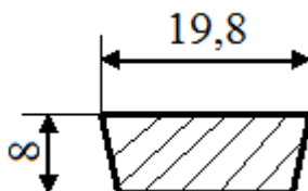
Рисунок 13 – Эскиз сечения питателя
