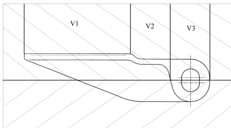
Рисунок 15 – Схема определения воображаемых столбов формовочной смеси
