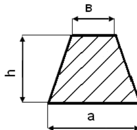
Рисунок 6 – Эскиз сечения шлакоуловителя
