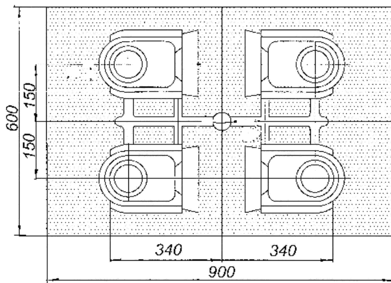
Рисунок 2 – Схема расположения отливок в литейной форме
