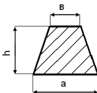
Рисунок 3 – Эскиз шлакоуловителя
