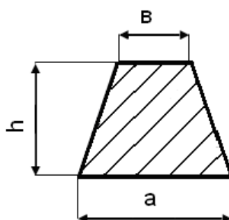
Рисунок 11 – Эскиз сечения литникового хода
