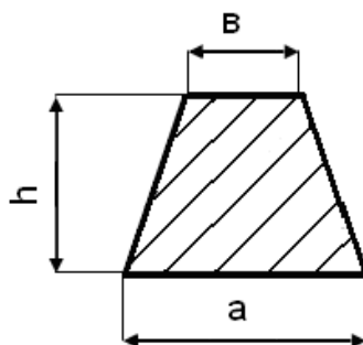
Рисунок 3 – Эскиз шлакоуловителя
