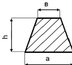
Рисунок 9 – Эскиз сечения литникового хода
